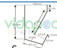
C Comedero para jaula de conejo
